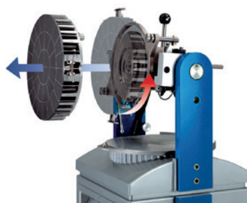
Disco divisor intercambiable.
